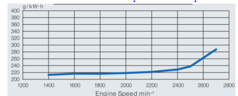
Biểu đồ tiêu thụ nhiên liệu
