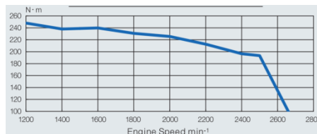
Biểu đồ Momen xoắn
