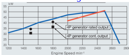
Biểu đồ công suất
